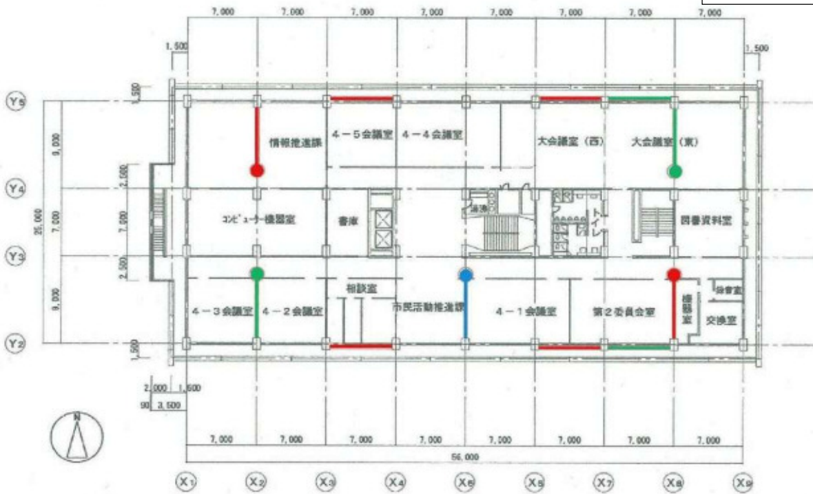
4階平面図
