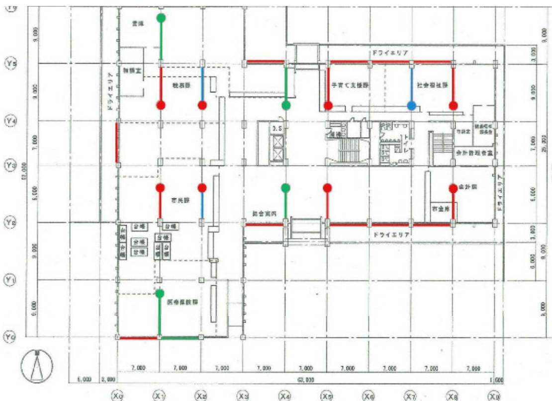
1階平面図
