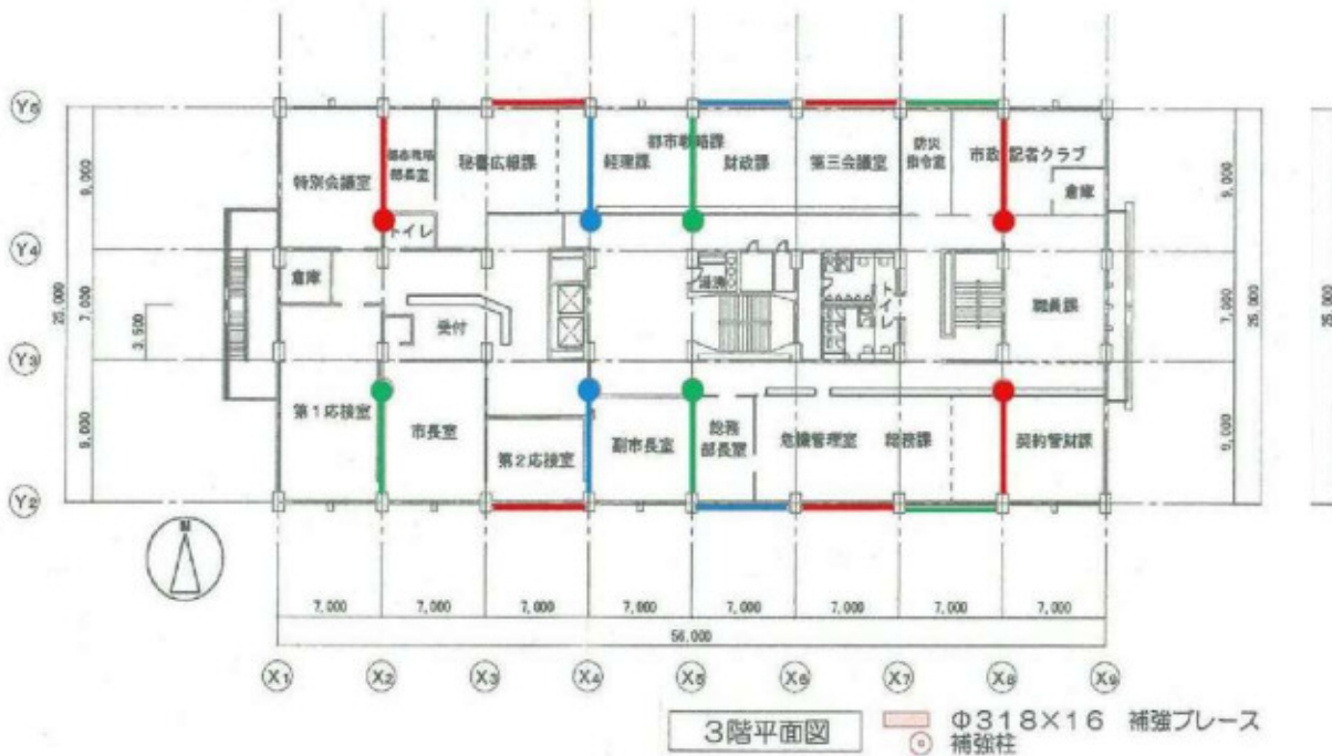
3階平面図
