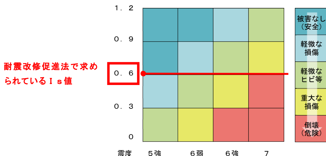
図 I-4. 2 I s 値と地震による被害想定
